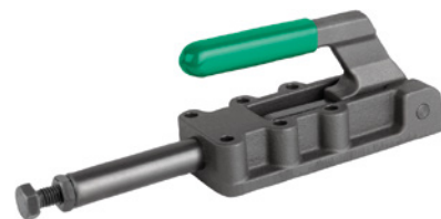
05840 Sauterelle à pousser et tirer modèle lourd avec poignée
