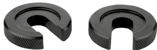
07420 Rondelle concave, rondelle convexe DIN 6319, 10/01
